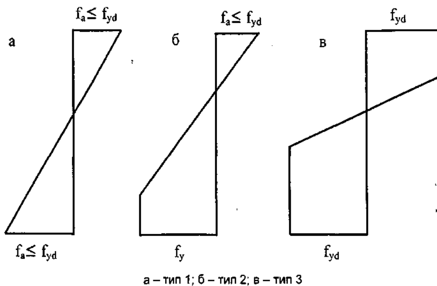
Рисунок 9.2 - Типи напружено-деформованого стану перерізу сталевго профілю сталезалізобетонних балок
