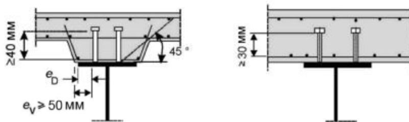
Рисунок 9.3 — Деталювання
