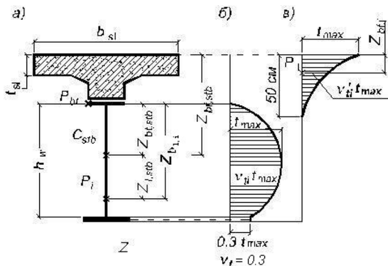
а - схема поперечного перерізу; б - криволінійна епюра розподілу температур по висоті сталеві частини перерізу; в - криволінійна епюра розподілу температур для верхньої частини перерізу балки
