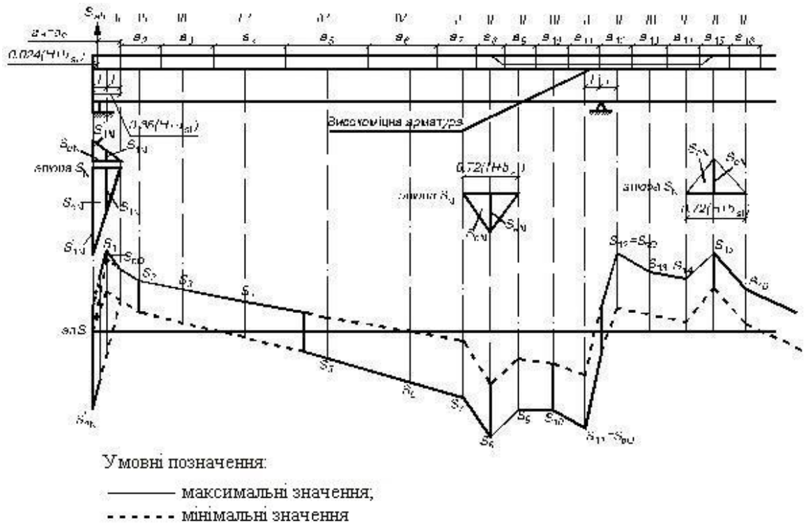
Рисунок Г.1 – Епюри погоних зсувних сил між залізобетонною та сталевією частинами I, II, III, IV – розрахункова довжина ділянок a_i
