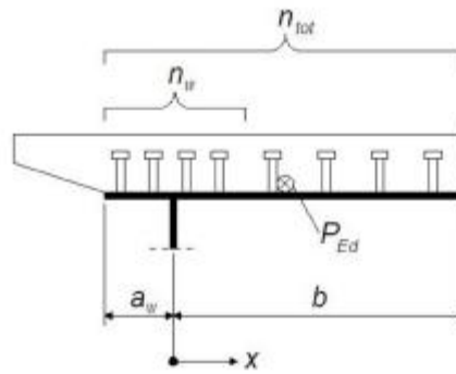
Рисунок 9.5 – Визначення позначень за рівнянням (9.8)
