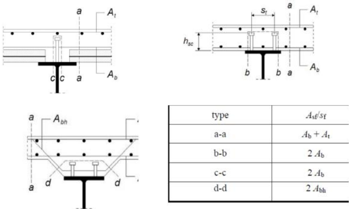
Рисунок 9.4 – Типові потенційні поверхні руйнування при зсуві
