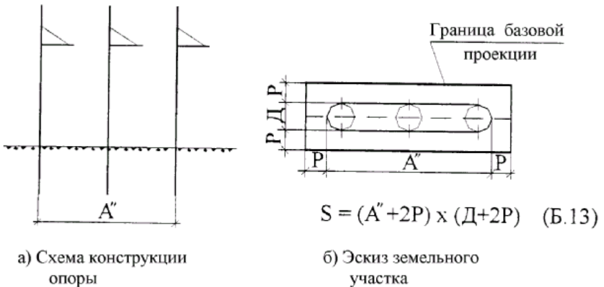
Рисунок Б. 12 - Опора из трех отдельных стоек
